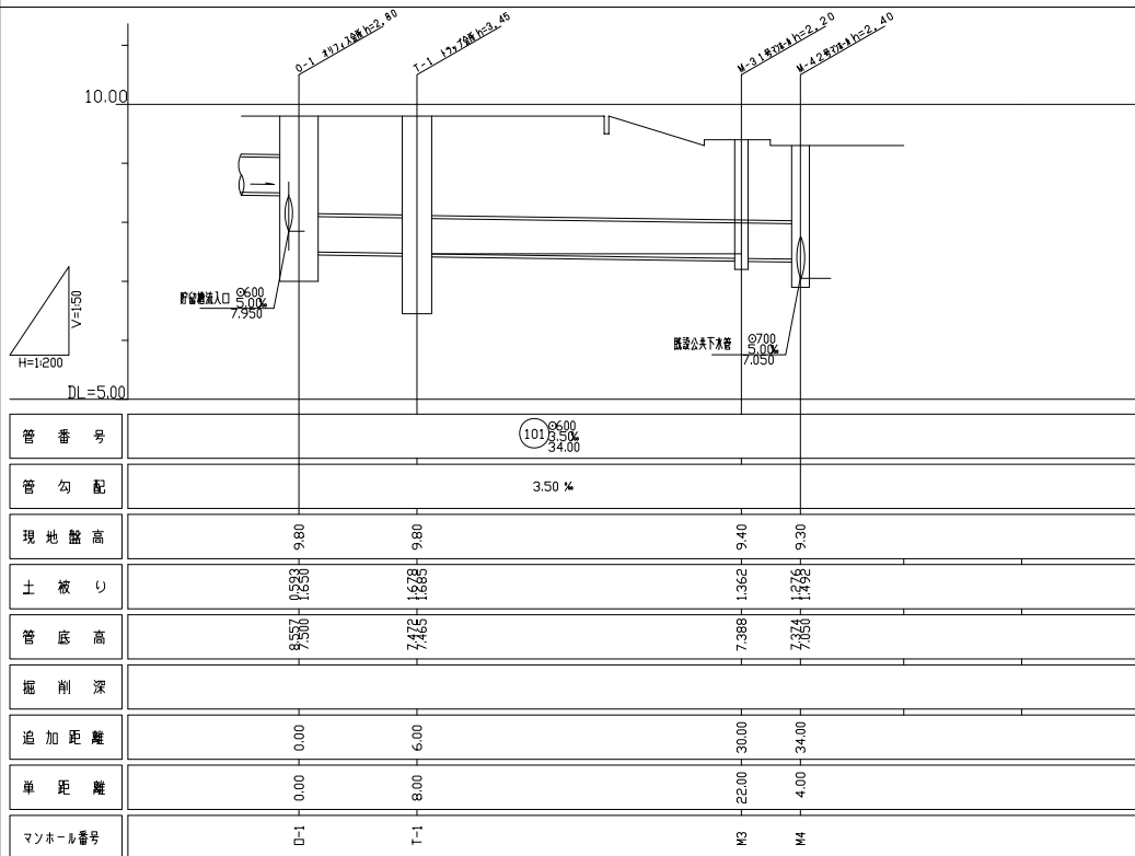
放流先縦断図
